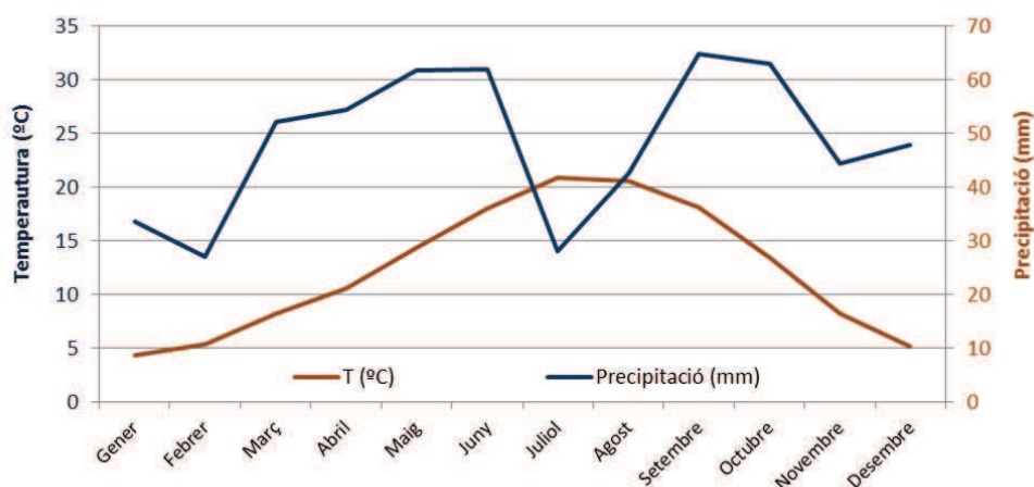
Figura 1. Diagrama ombromètric de Calaf. Mitjana de 1953-1980. / Font: Caracterització agroclimàtica de la província de Barcelona. 1989. Ministerio de Agricultura, Pesca y Alimentación.
